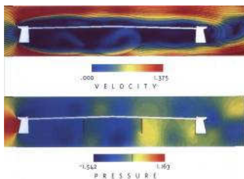
Fig. 2 – Estudos aerodinâmicos
