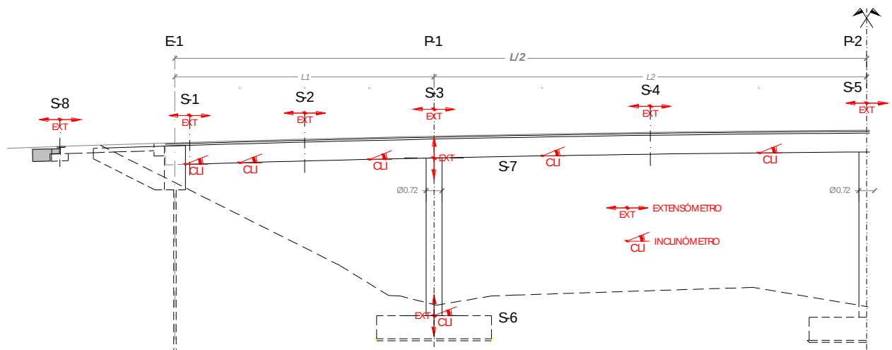
Figura 2: Esquema de instrumentación. Vista Lateral de la mitad instrumentada del puente.
