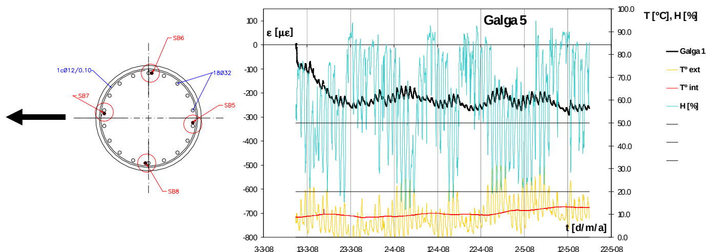
Figura 9: Deformaciones experimentales de la sección de la Pila, en la galga nº 5. Registro de deformaciones, temperatura y humedad en obra.
